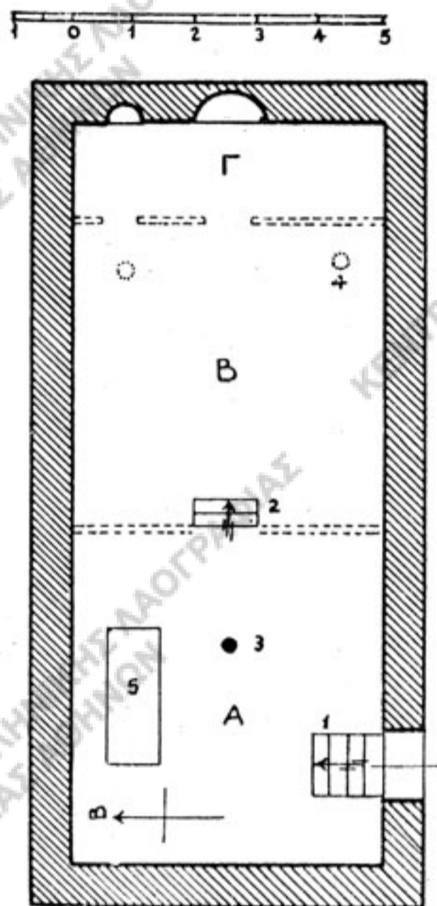
Εἰκ. 14. — Κάτοπις ναοῦ Ἁγίου Ἀθανασίου Μεταξάδων.
