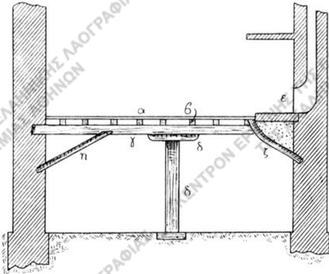
Εἰκ. 16.— Τομὴ δαπέδου ἀνωγείου - ὀροφῆς κατωγείου.
