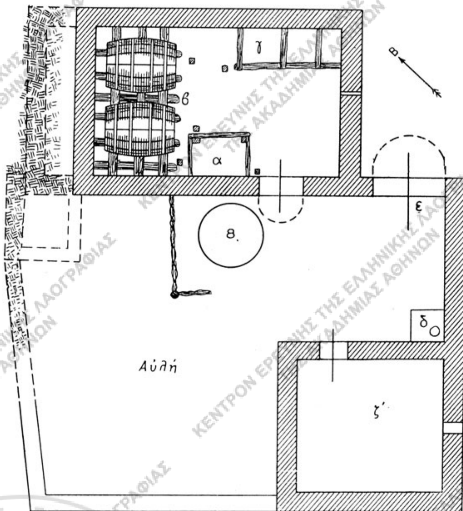
Εἰκ. 1. — Κάτωρις κατογείου καὶ αὐλῆς τῆς οἰκίας Στ. Γκίκα.
