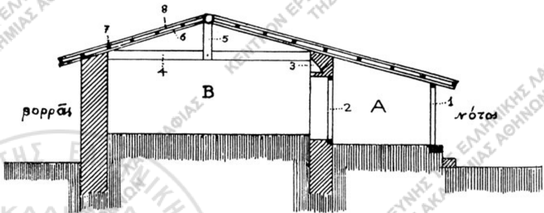
Εἰκ. 1. — Κάτοψις καὶ κατὰ πλάτος τομὴ παλαιᾶς οἰκίας τοῦ χωρίου Τριφύλλι.
