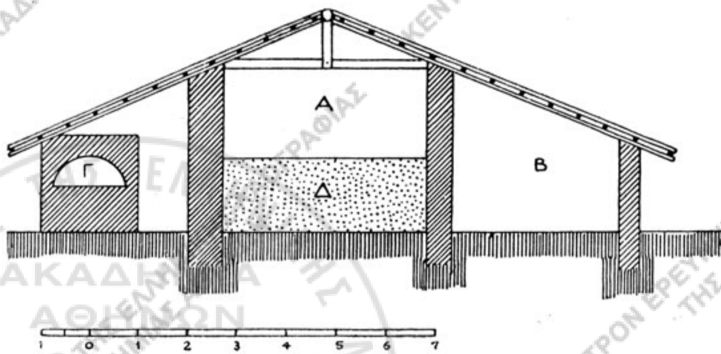
Εἰκ. 23. - Κάτωρις καὶ κατὰ μῆκος τομὴ οἰκίας Α τοῦ χωρίου Παλιούρι.
