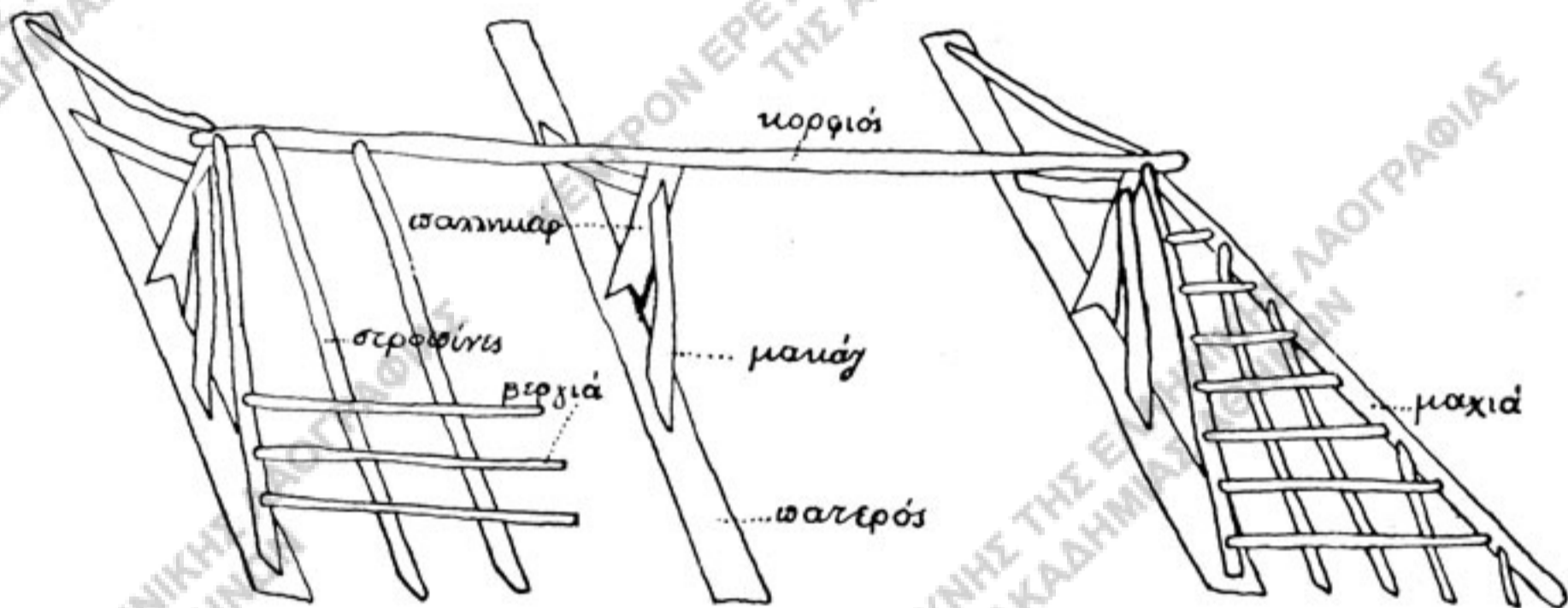
Εἰκ. 18. - Ὀνοματολογία στέγης 2) .
