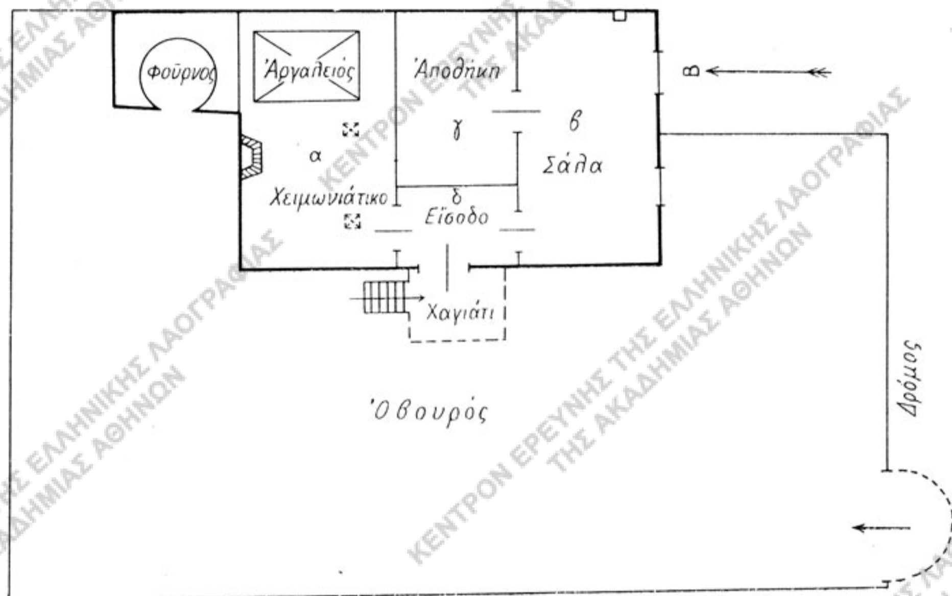
Εἰκ. 10. — Σχέδιον οἰκίας Εὐστ. Βελόνη.
