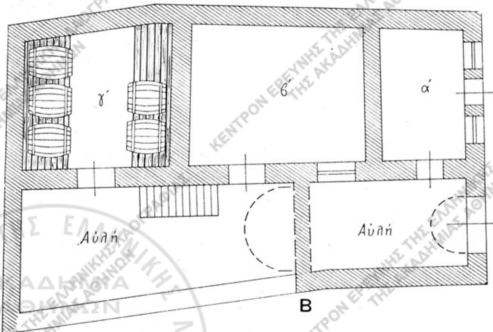
Εἰκ. 12. — Κάτοπις οἰκίας Α. Μπακάλη.
