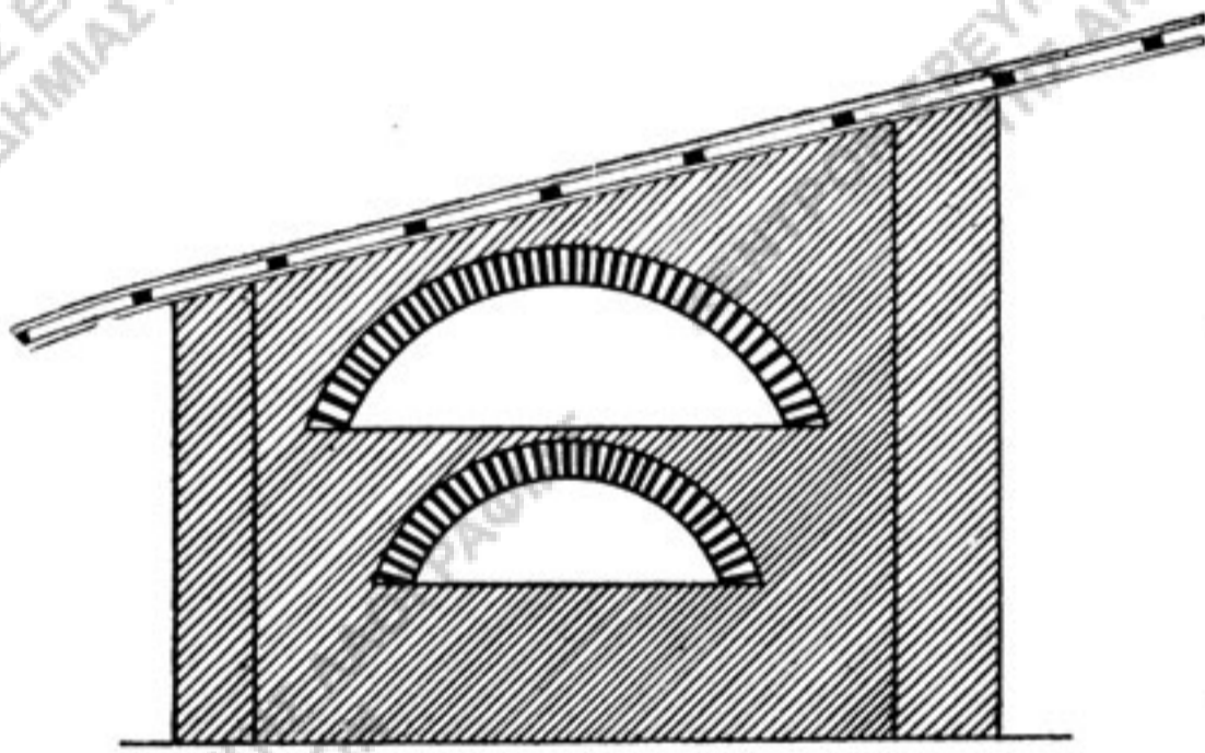
Εἰκ. 12. - Διπλοῦς φοῦρος.
