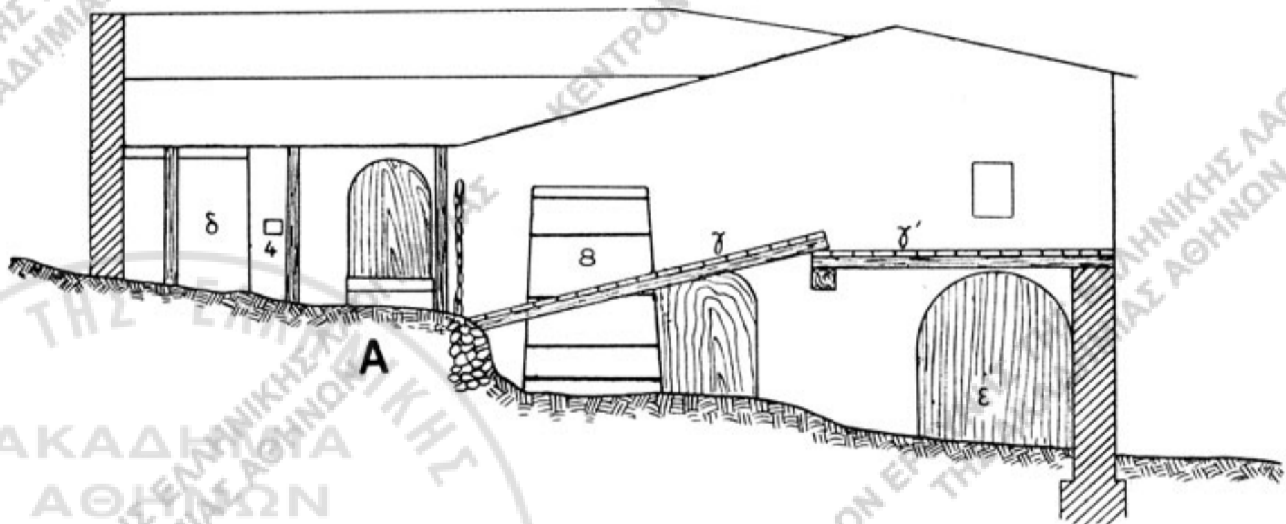
Εἰκ. 2. — Κάτοπις ἀνογείου καὶ τομὴ κάθετος οἰκίας Γκίζα.
