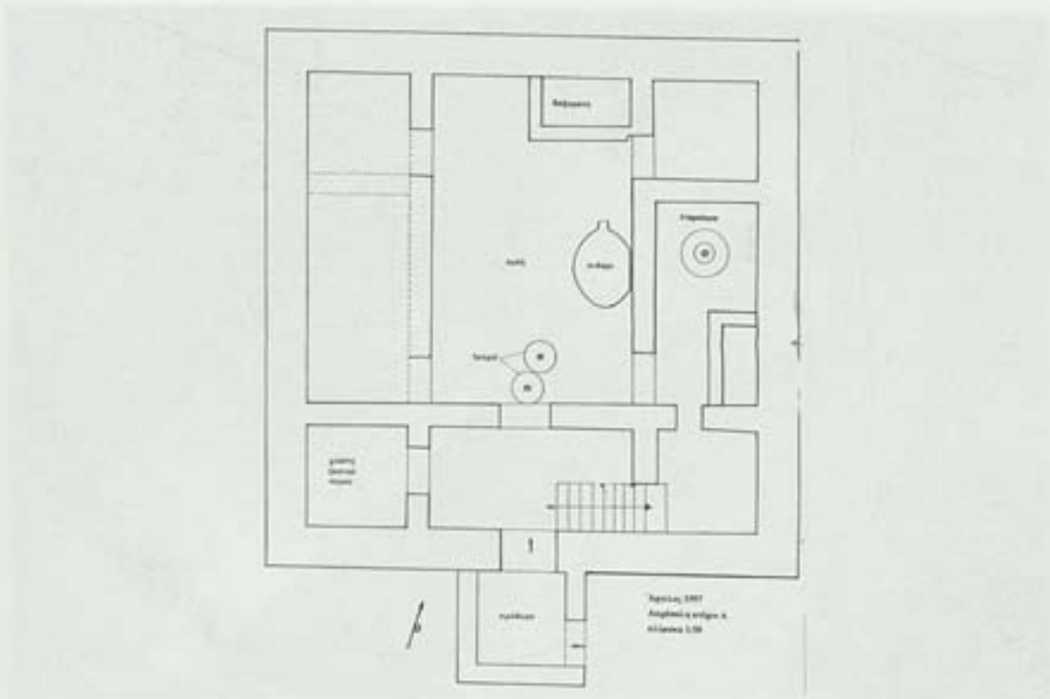
Σχέδιο 1. Κάτοψη του κτηρίου Α (ελαιουργείου).
