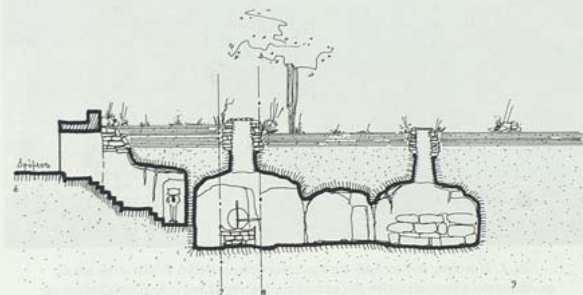
Σχ. 3. Κατακόρυφη τομή κατά τη διεύθυνση 6, 7, 8, 9.
