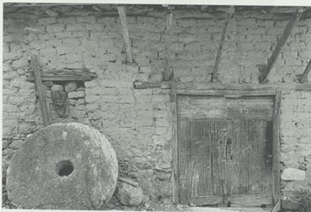
Εικ. 4. Ιπποκίνητο ελαιοτριβείο (Βουνάρια Μεσσηνίας, 1998).
